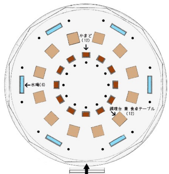
炊飯棟平面図（A～Cサイト）
